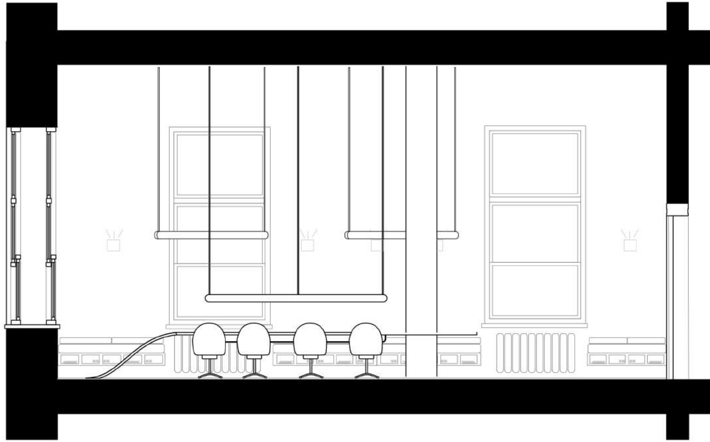
B KESİTİ
